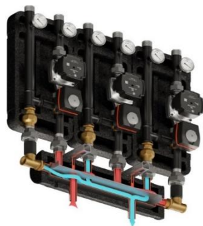
Brygada 3D+ pionowe z odpływami w dół
